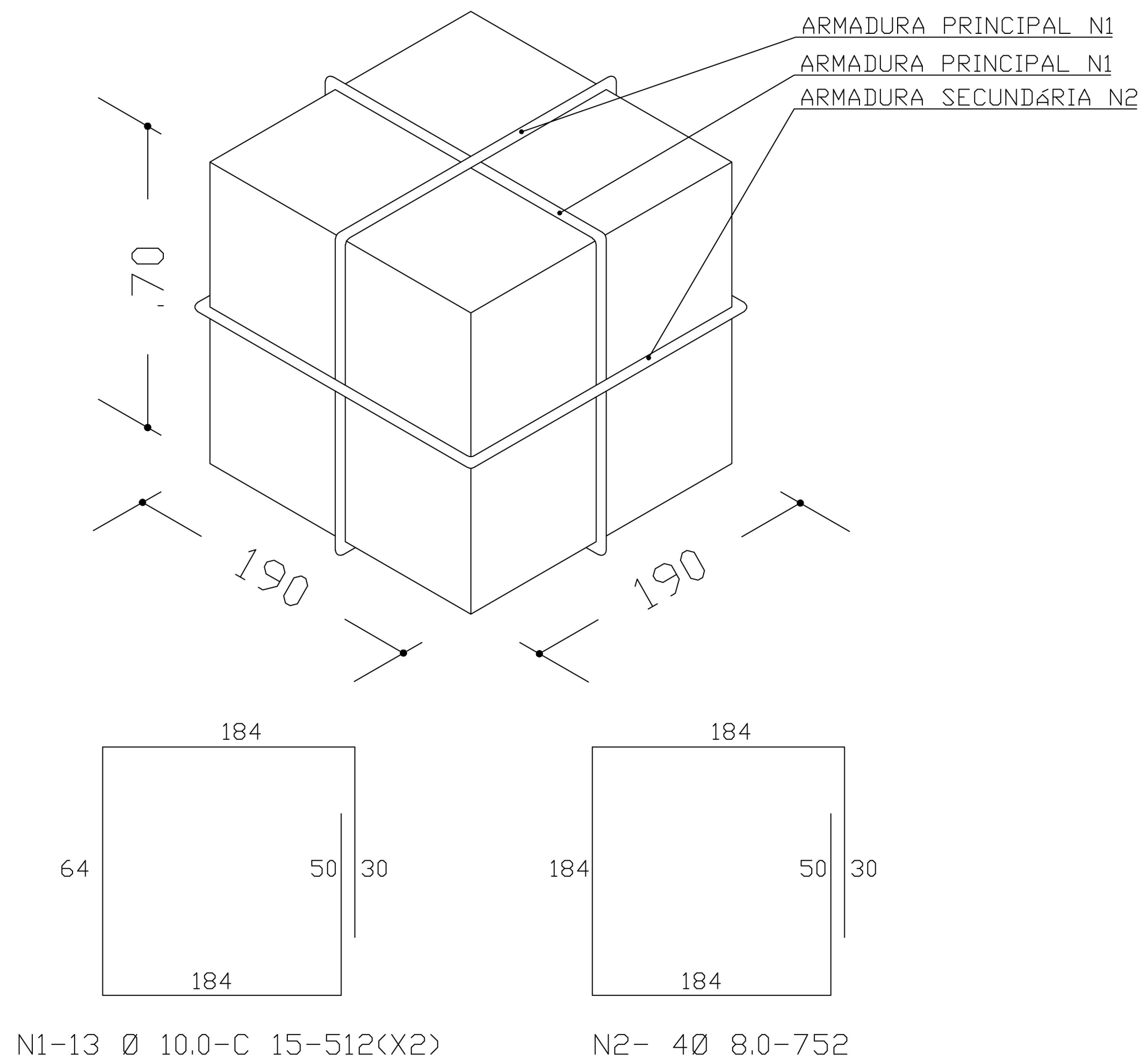
ARMADURA DO BLOCO P/ CX. 5000L SEM ESCALA
